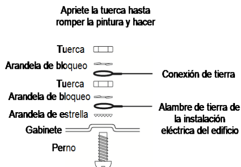
Figura 2-18 Instalación de tierra
