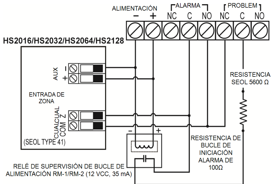
Figura 2-17 Cableado del detector de CO
