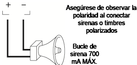
Figura 2-13 Cableado de terminales sirena
