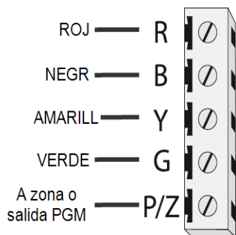
Figura 2-8 Terminales del teclado
