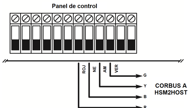
Figura 2-6 Diagrama de cableado del HSM2HOSTx
