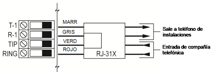
Figura 2-14 Cableado de línea telefónica
